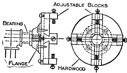
Fig. 4—Chuck
