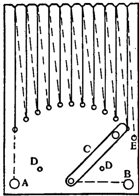
Battery Rheostat
