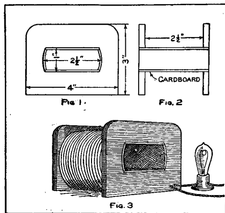
Watch Demagnetizer
