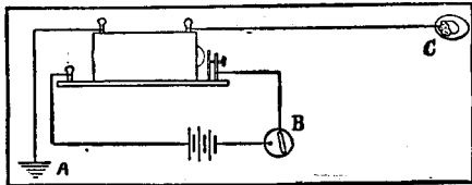
Shocking-Machine
