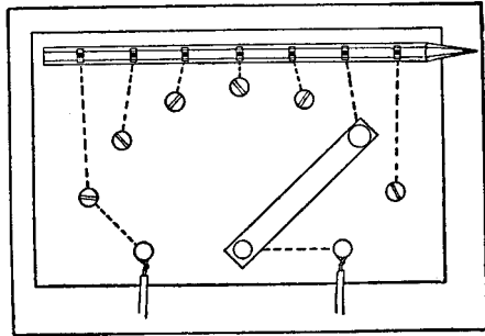
Simple Rheostat
